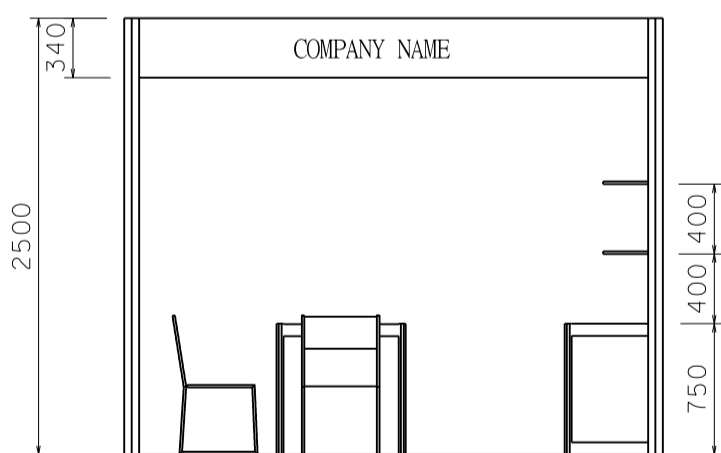
ELEVATION 正面圖
