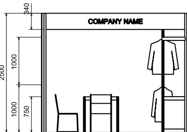
ELEVATION 正面圖
